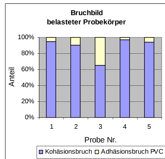
Diagramme 3 und 4 Grafische Darstellung der Bruchbilder unbelasteter Probekörper und mechanisch belasteter Probekörper.
