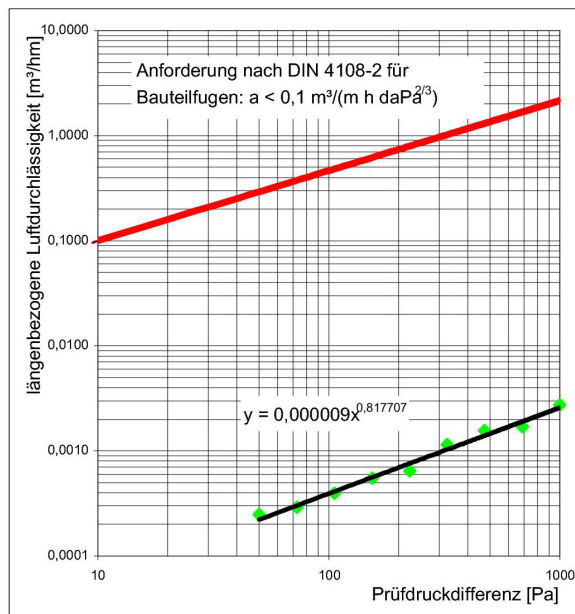
Grafik 2 Längenbezogene Luftdurchlässigkeit Q
