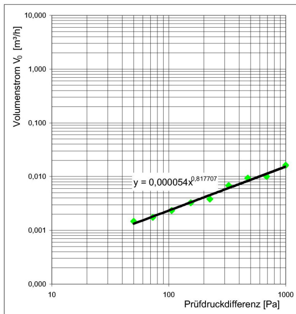
Grafik 1 Volumenstrom V_0
