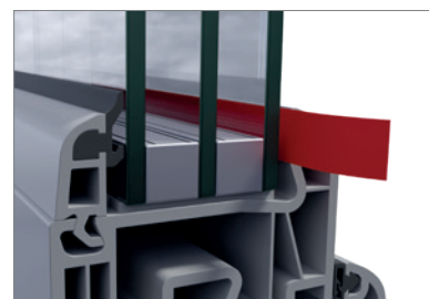
Direktverglasungen
